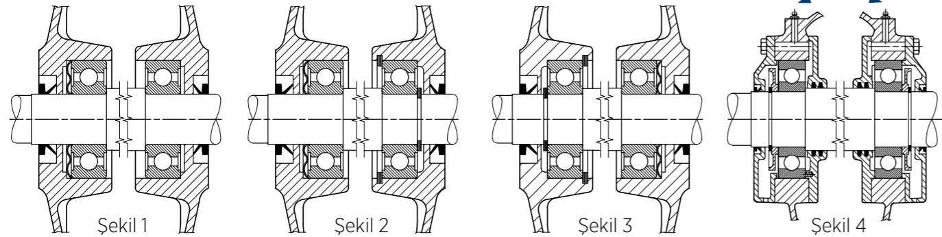
Ön Serbest yatak (Yay gerilmeli) Arka Serbest yatak Ön Serbest yatak (Yay gerilmeli) Arka Sabitlenmiş yatak Ön Sabitlenmiş yatak Arka Serbest yatak (Yay gerilmeli) Ön Serbest yatak (Yay gerilmeli) Arka Sabitlenmiş yatak
