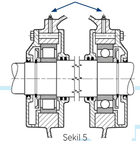
Ön Makaralı rulman Arka Sabitlenmiş yatak Şekil 5
