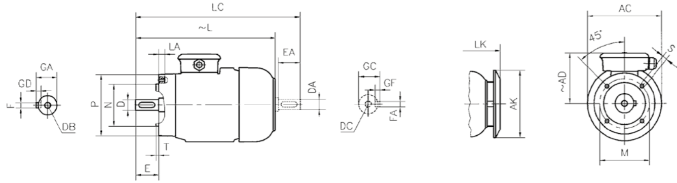
Flanşlı motor boyutları: (Flanş biçimi C- DIN EN 50 347) B14, V18, V19 yapı biçimlerinde
