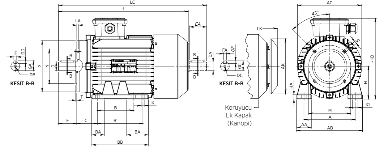
Ayaklı ve flanşlı motor boyutları: (Flanş biçimi C- DIN EN 50 347) B34 yapı biçiminde
